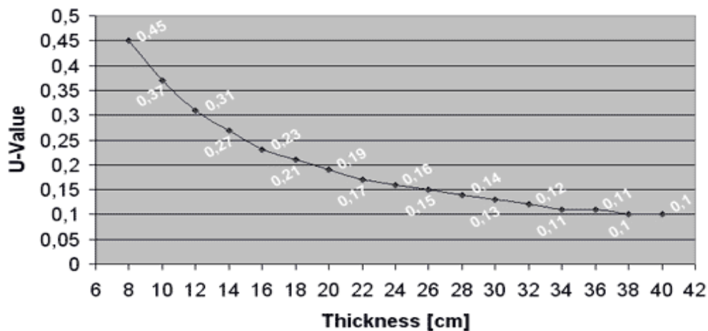
Thermofloc - U-Value
